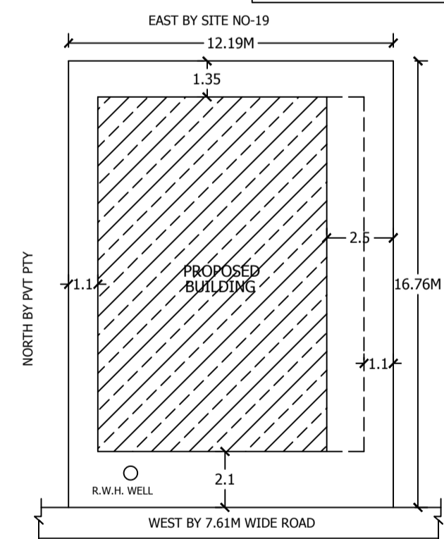
SITE PLAN 1:200
